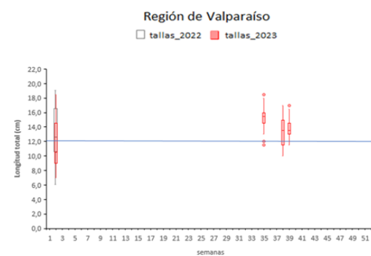
b) Anchoqueta
